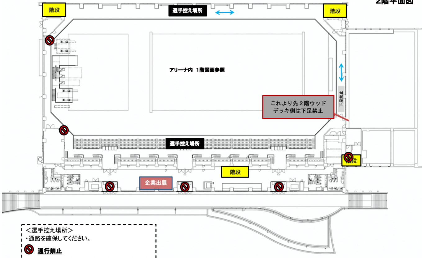
2階平面図
